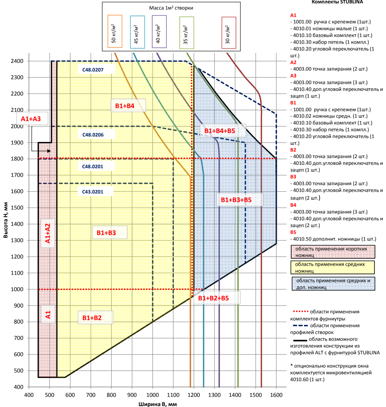
График для выбора размеров п/о створки и комплектов фурнитуры STUBLINA 4010.00 (комплект петель для нагрузки до 100 кг) для конструкций ALT C43 и ALTC48
