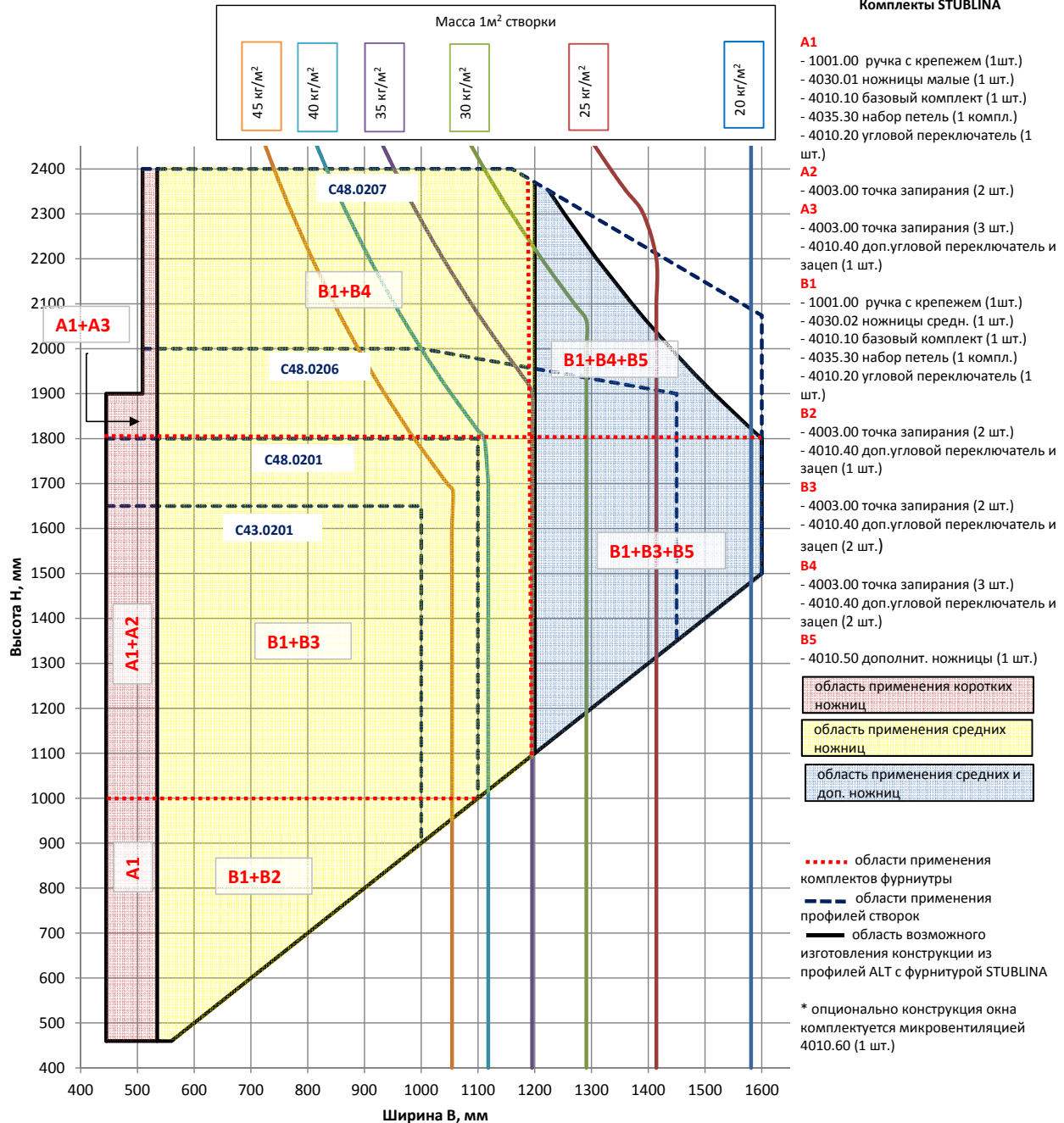
График для выбора размеров п/о створки и комплектов фурнитуры STUBLINA 4030.00 (комплект петель для нагрузки до 80 кг) для конструкций ALT C43 и ALTC48
