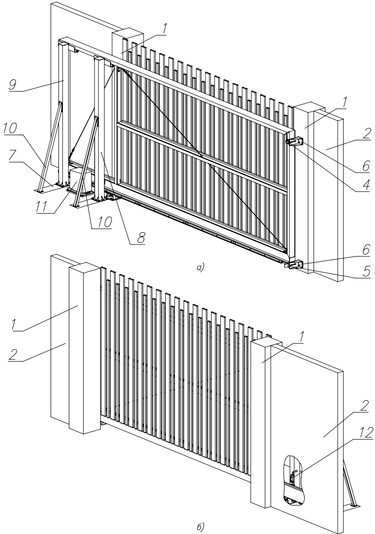
Мал. 1. Відкотні самонесучі ворота з накладним вертикальним розрідженим заповненням алюмінієвими профілями, відкриття вліво а — вигляд з боку двору, б — вигляд з боку вулиці
