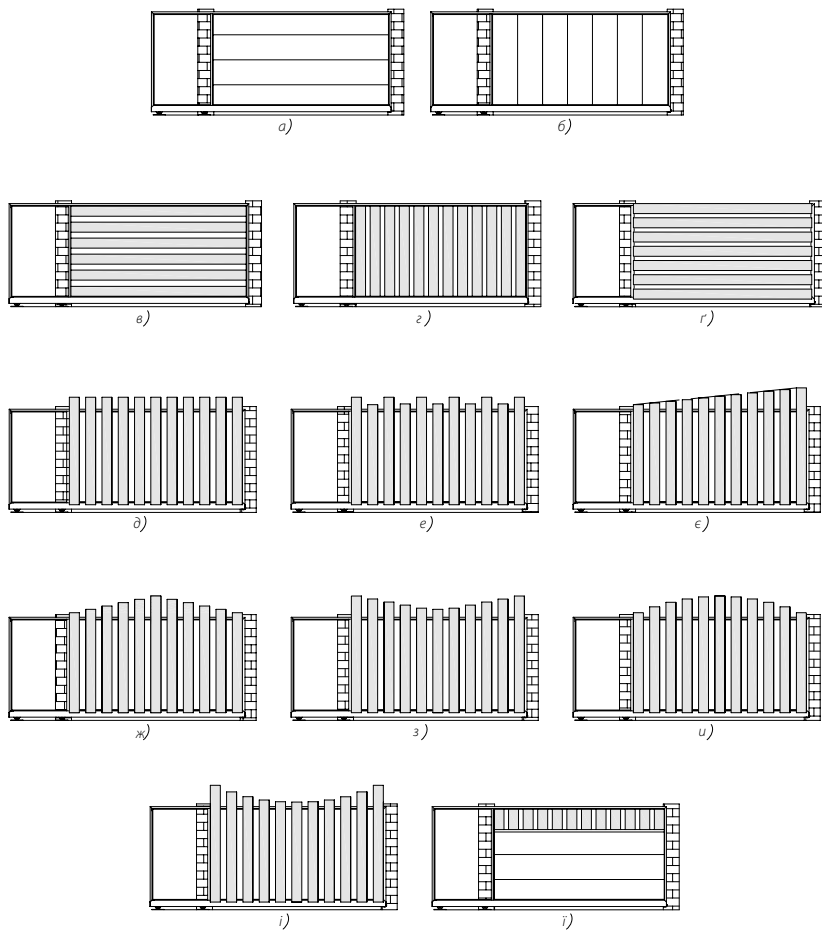
Мал. 2. Схематичні зображення видів монтажу заповнення
